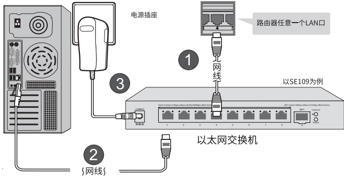
图4-1 交换机连接线缆示意图
